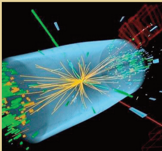
Foto: CMS/CERN
